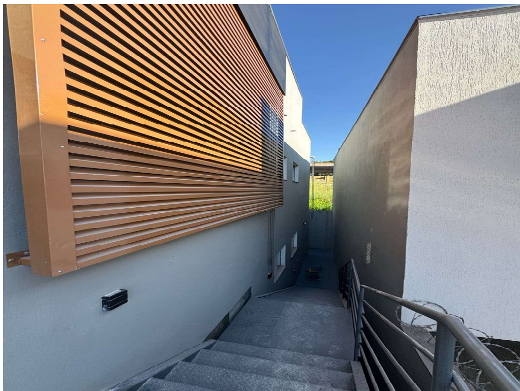
FOTO 46 - EXECUÇÃO DE ESCADA. INSTALAÇÃO DE BRISE E PÓRTICO METÁLICO. EXECUÇÃO DE PINTURA. INSTALAÇÃO DE ARANDELAS E REFLETORES.
