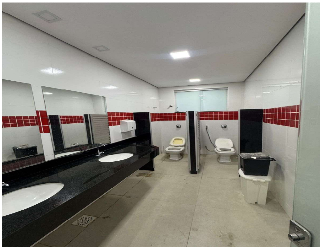
FOTO 21 - EXECUÇÃO DE FORRO EM GESSO. EXECUÇÃO DE PINTURA. INSTALAÇÃO DE LUMINÁRIAS. INSTALAÇÃO DE ACABAMENTO DE VÁLVULA.
