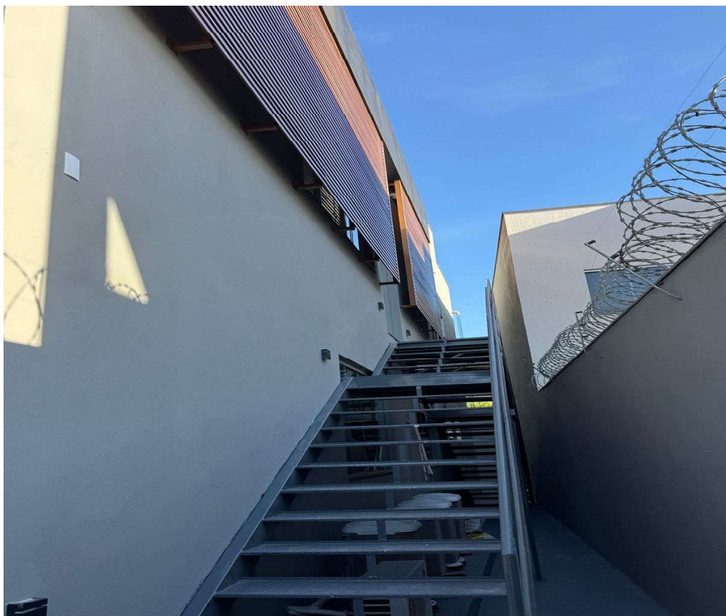
FOTO 47 - INSTALAÇÃO DE BRISE E PÓRTICO METÁLICO. EXECUÇÃO DE PINTURA. INSTALAÇÃO DE ARANDELAS E REFLETORES.
