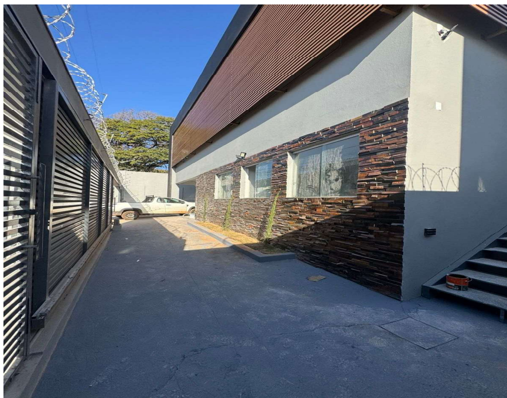
FOTO 48 - INSTALAÇÃO DE BRISE E PÓRTICO METÁLICO. INSTALAÇÃO DE PEDRA FERRO. EXECUÇÃO DE PINTURA. INSTALAÇÃO DE REFLETORES. PINTURA DE PISO. EXECUÇÃO DE CANTEIRO E JARDIM.
