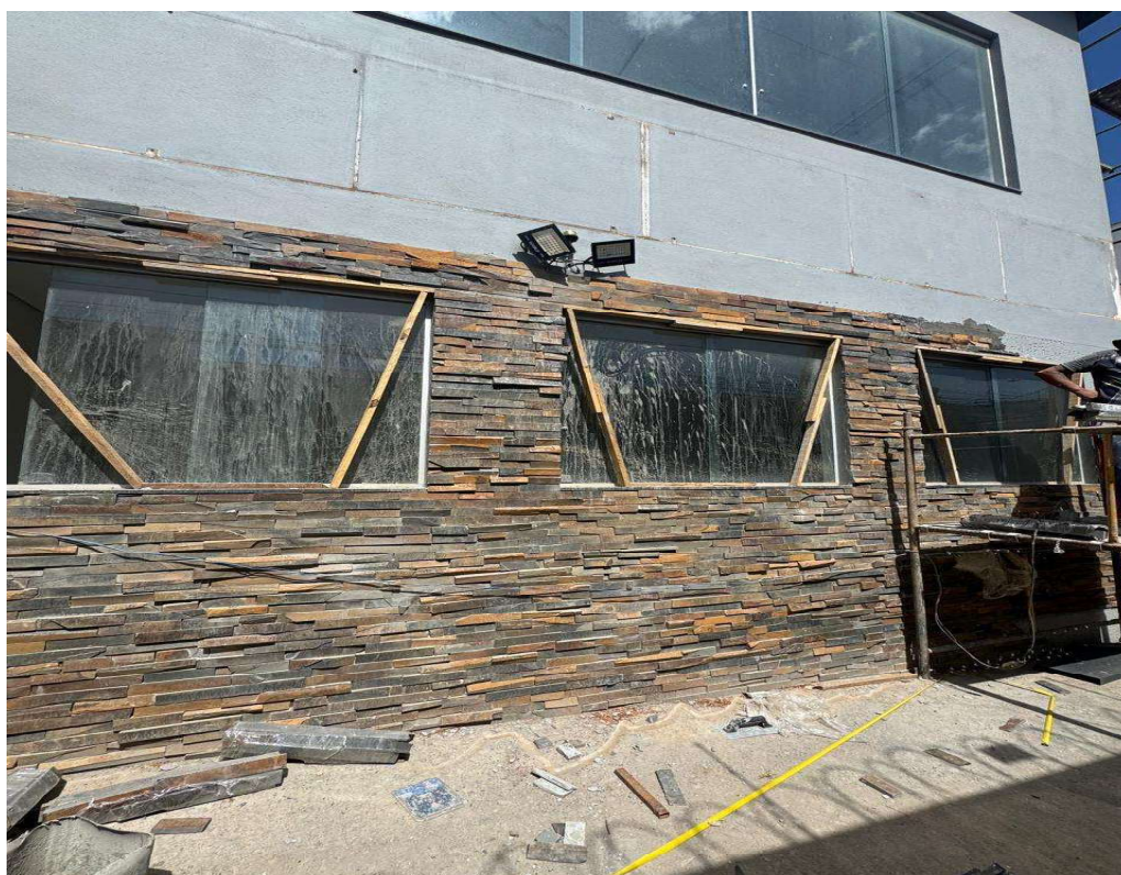
FOTO 14 - INSTALAÇÃO DE PEDRA FERRO.
