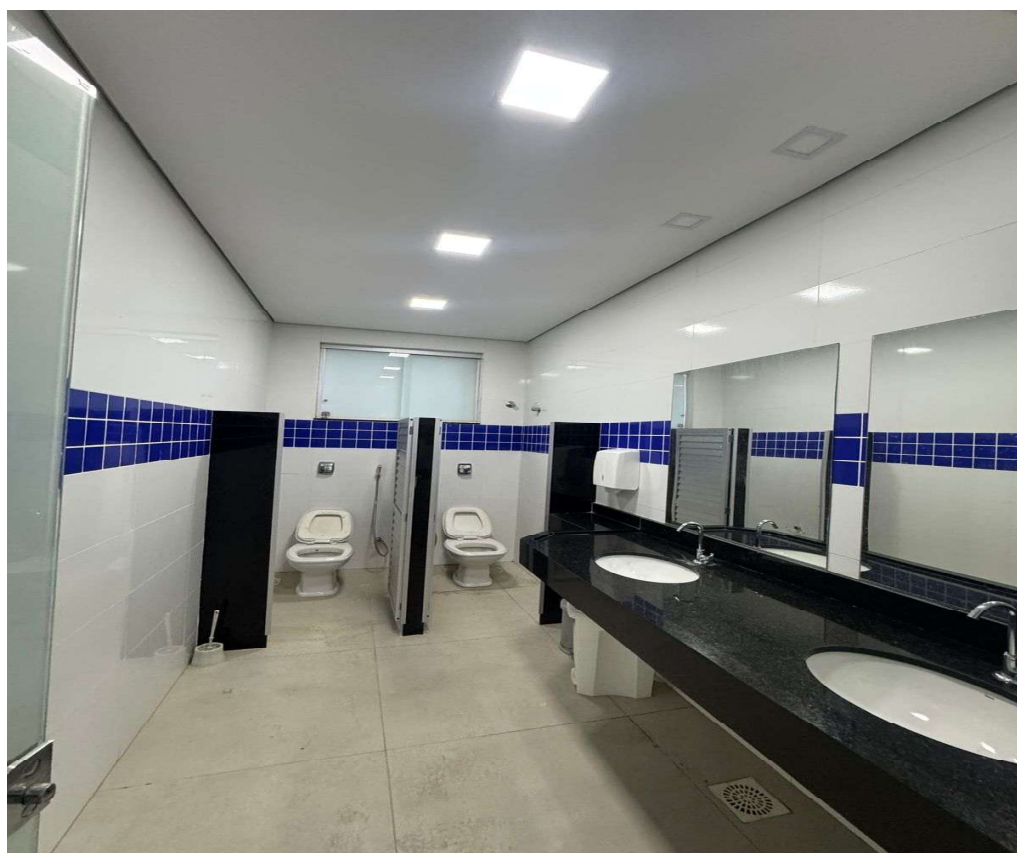
FOTO 22 - EXECUÇÃO DE FORRO EM GESSO. EXECUÇÃO DE PINTURA. INSTALAÇÃO DE LUMINÁRIAS.
