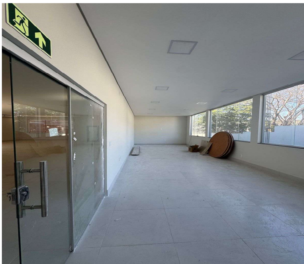
FOTO 38 - EXECUÇÃO DE FORRO EM GESSO E PAREDES DE DRYWALL - FOI REALIZADA A ADEQUAÇÃO DA PAREDE EM SISTEMA DRYWALL COM INSERÇÃO DE REFORÇOS INTERNOS NA ESTRUTURA, DIMENSIONADOS PARA RECEBER A FIXAÇÃO DOS MÓVEIS PLANEJADOS. ASSENTAMENTO DE PISO E RODAPÉ. EXECUÇÃO DE PINTURA. INSTALAÇÃO DE AR-CONDICIONADO. INSTALAÇÃO DE LUMINÁRIAS, TOMADAS E INTERRUPTORES. INSTALAÇÃO DE PORTA. INSTALAÇÃO DE PLACAS DE SINALIZAÇÃO.
